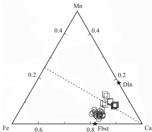
Рис. 7. Соотношения главных M -катионов в: □ — дальнегорските из Дальнегорского месторождения (данная работа) и месторождения Хидзиказу, Япония (Ohashi, Finger, 1978), и ○ — ферробустамите (Rapoport, Burnham, 1973; Shimazaki, Yamanaka, 1973; Burnham, 1975; Yamanaka et al., 1977; Шипалкина и др., 2018). Звездочками обозначены составы гипотетических конечных членов дальнегорскита (Dln) и ферробустамита (Fbst).
