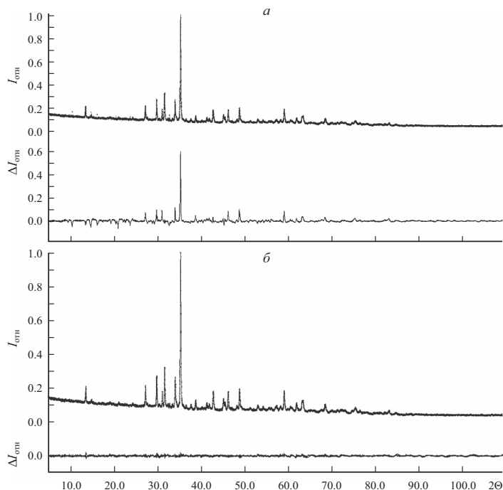
Рис. 6. Результаты уточнения кристаллической структуры дальнегорскита методом Ритвельда с использованием моделей волластонита ( a ) и бустамита ( б ). Для каждого рисунка: верхний график — экспериментальная порошковая дифрактограмма дальнегорскита, нижний график — разностная кривая интенсивностей экспериментальной и расчетной рентгенограмм.
