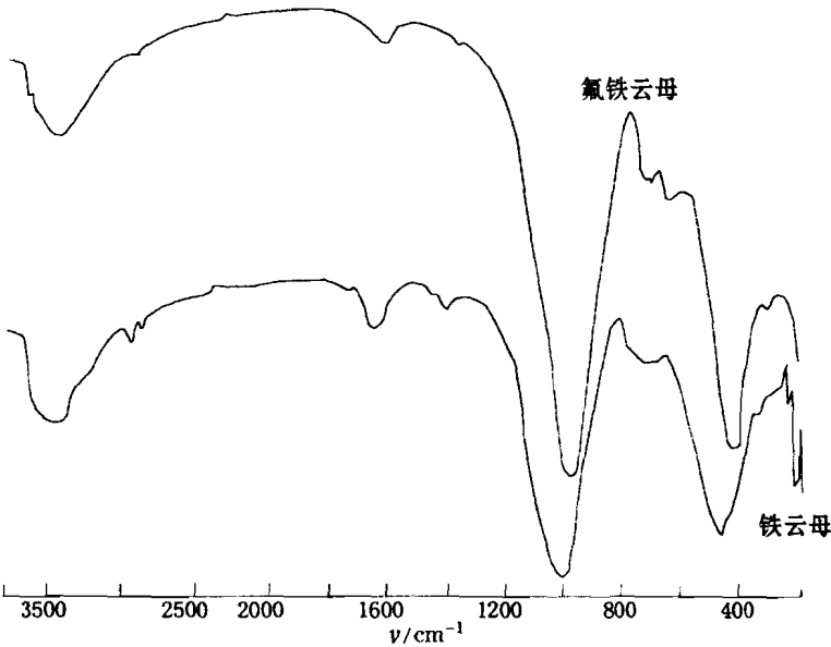
图 1 氟铁云母和黄山铁云母的红外光谱
