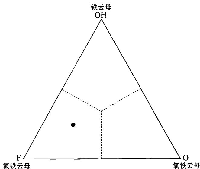
图2 不同附加阴离子成分的铁云母端员矿物分类命名图
