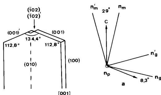
FIG. 2. — Macule de françoisite-(Nd) avec les principaux angles et l'orientation optique. Plan de macule : (100).
