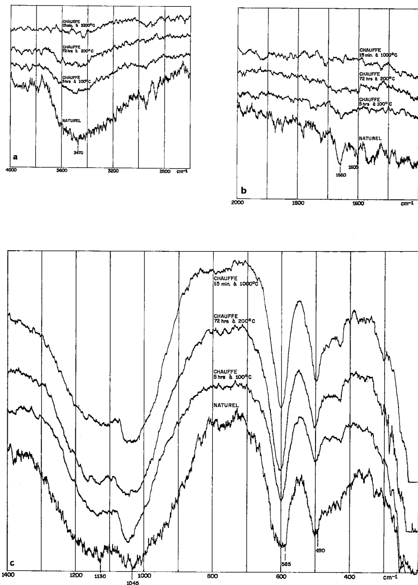
FIG. 2. Spectres d'absorption infra-rouge pour l'ekanite naturel et chauffé : (a) région de 4000 à 2700 \text{cm}^{-1} (b) région de 2000 à 1400 \text{cm}^{-1} (c) région de 1400 à 200 \text{cm}^{-1} . Noter la bande d'absorption à 3470 \text{cm}^{-1} et les pics à 1660 et 1605 \text{cm}^{-1} ( \text{H}_2\text{O}^- ).
